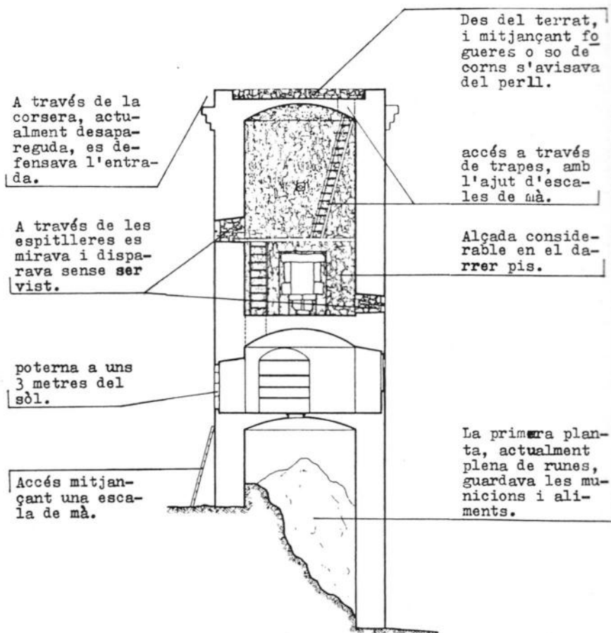
Secció de la Torre Valentina. Podem veure-hi algunes de les característiques esmentades anteriorment. Dibuix de l'autor.
